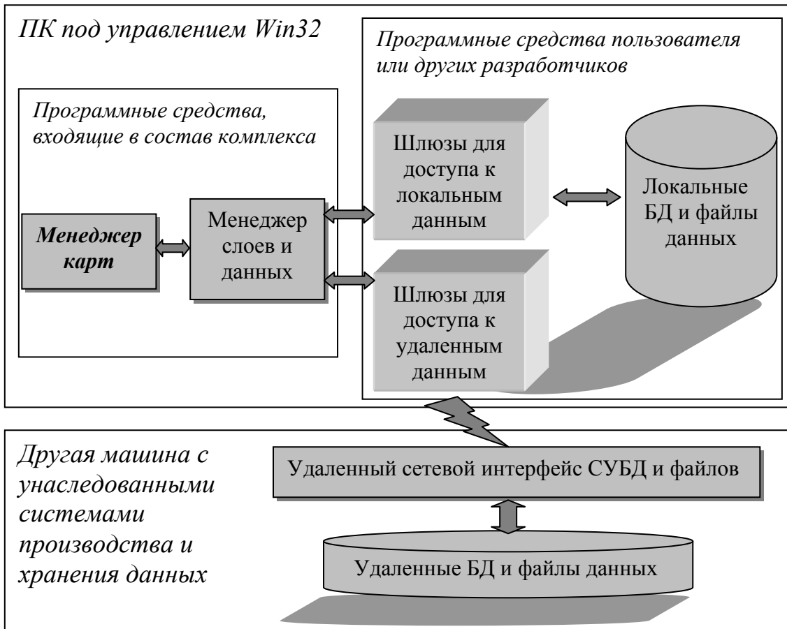
Рис. 2. Схема подключения данных пользователя к программе Isograh. Шлюзы для доступа к данным реализуются динамически загружаемыми библиотеками пользо-
