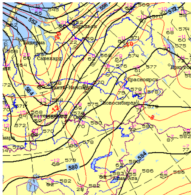
Рис. 2. Карта барической топографии поверхности 500 гПа за 12 ч ВСВ 5 июля 2021 г.
