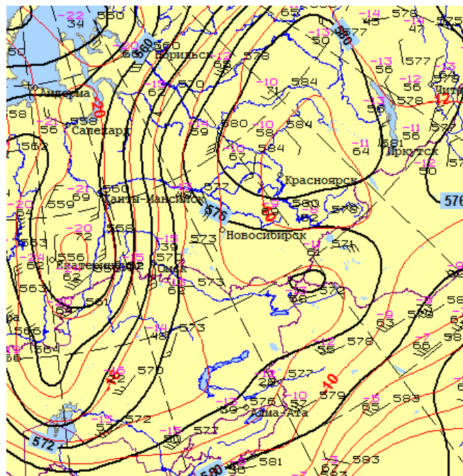
Рис. 1. Карта барической топографии поверхности 500 гПа за 12 ч ВСВ 1 июля 2020 г.
